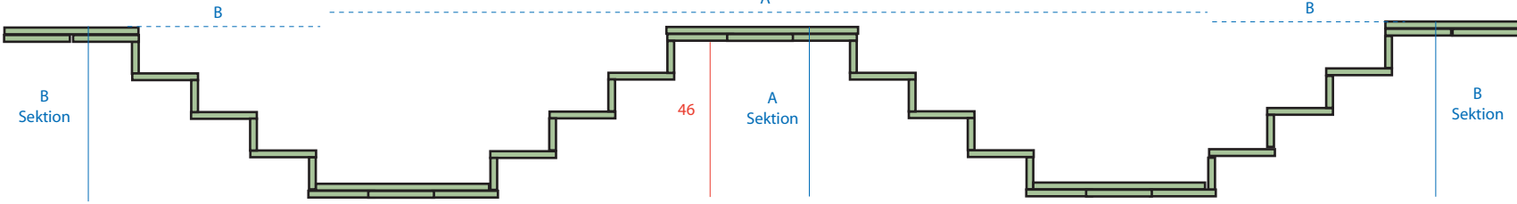
Sektion B, halvtätt plank
